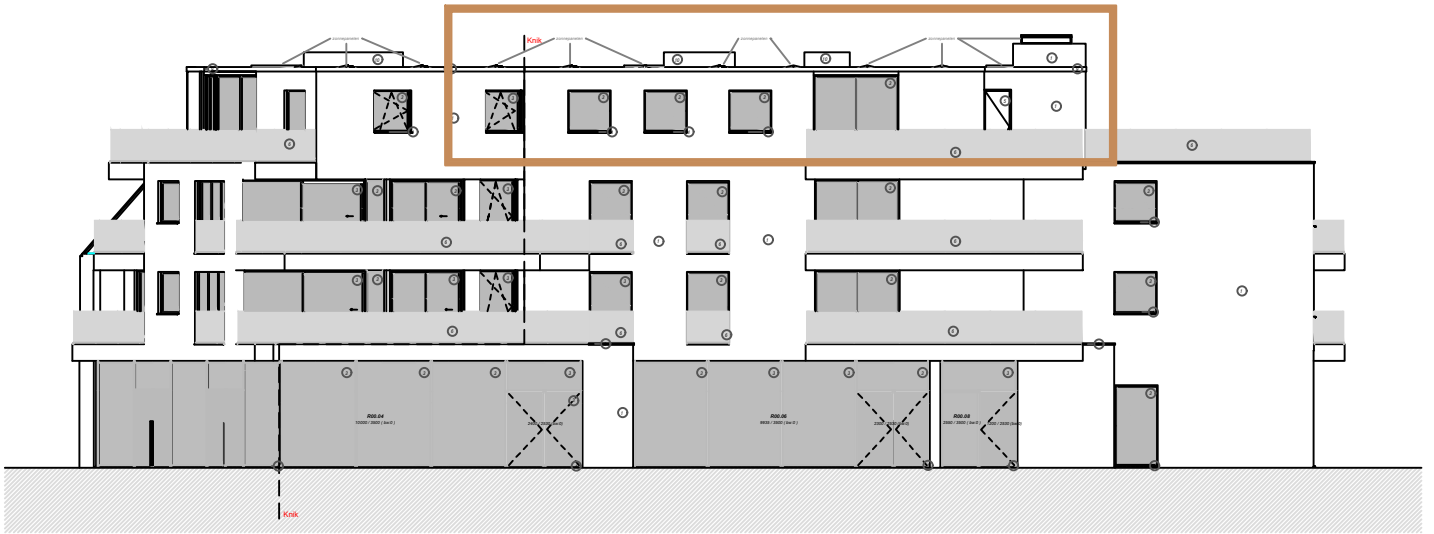
VOORGEVEL (NOORD)
