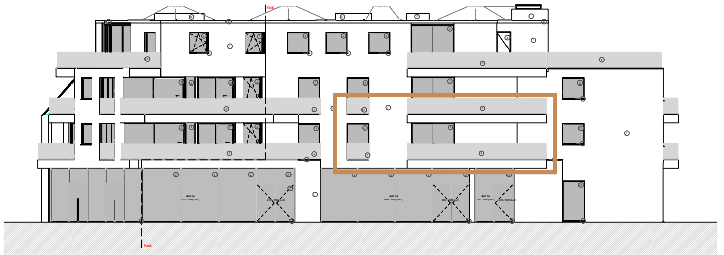
VOORGEVEL NOORD
